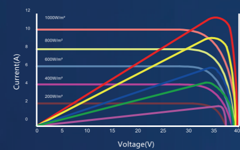
I-V Կոր
