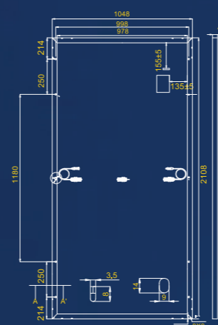
Ֆոտովոլտային մոդուլի չափերը
